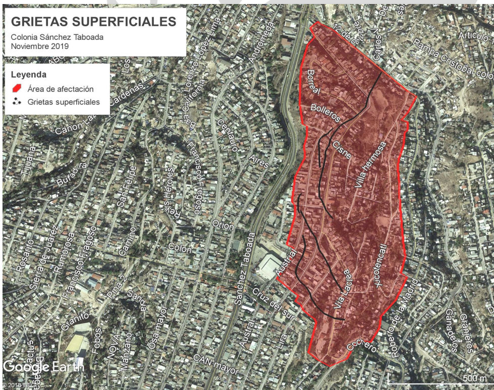
PLANO GENERAL. Agrietamiento superficial y zona de afectación.
